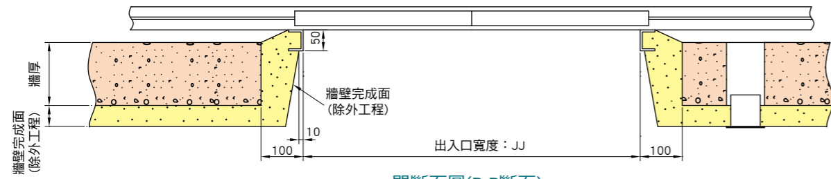
門斷面圖(B-B斷面)
