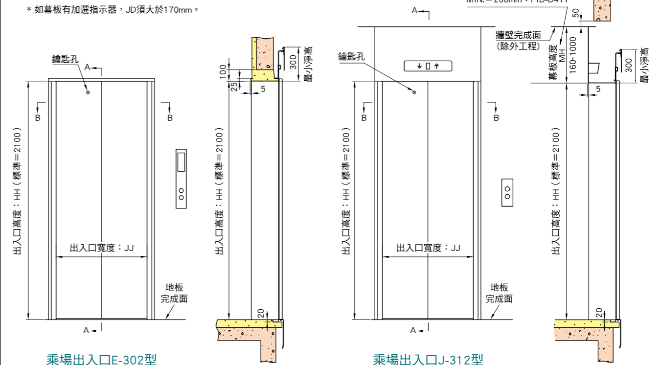
門斷面圖(A-A斷面)
