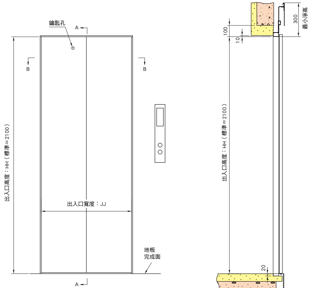
乘場出入口
