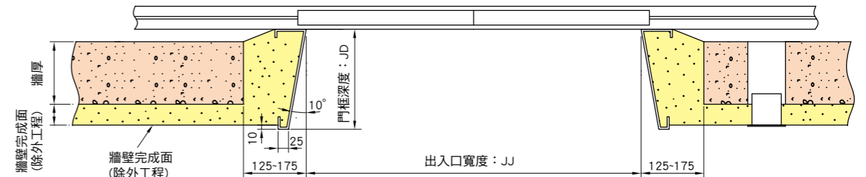
門斷面圖(B-B斷面)
